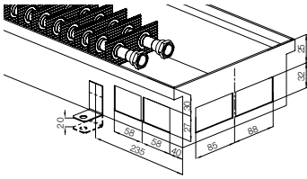
KORAFLEX FV
