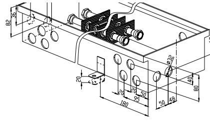
KORAFLEX FW 13/34
