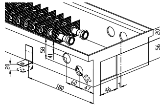
KORAFLEX FV 8/16
