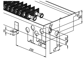
KORAFLEX FV 11/20
